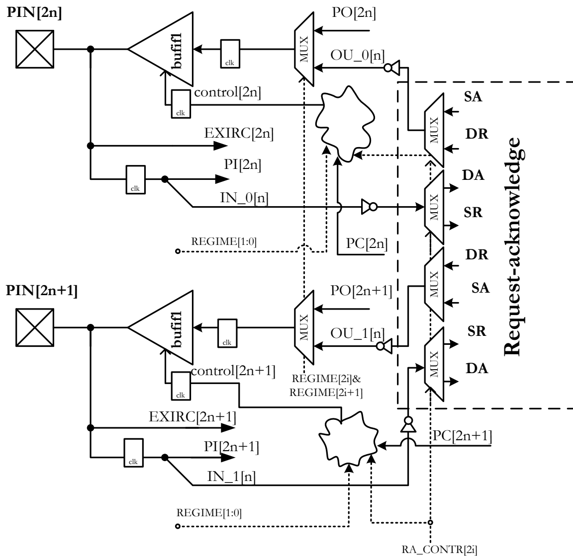
Рисунок 4.39 – Коммутация выводов интерфейсов, входящих в универсальный блок интерфейсов общего назначения
