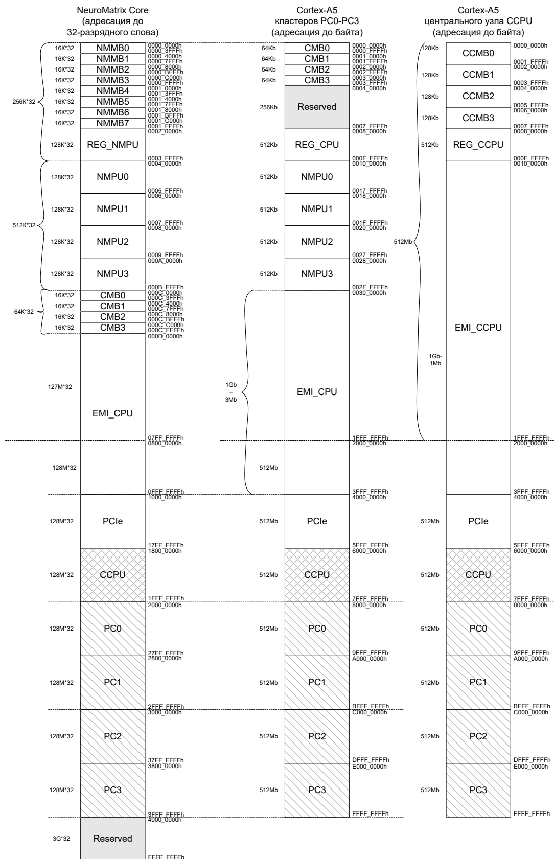
Рисунок 5.2 - Карта памяти микросхемы K1879BM8Я
