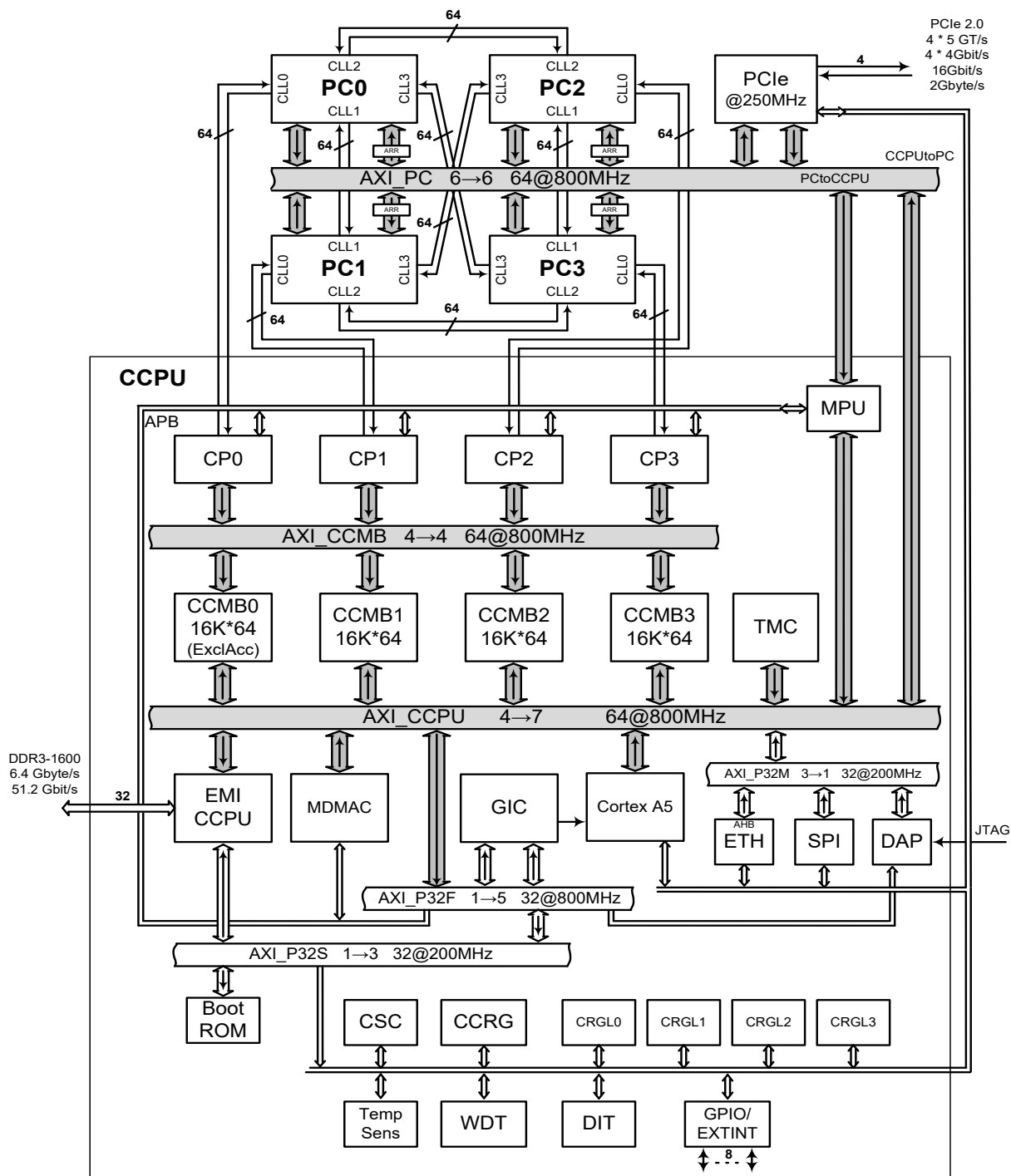
Рисунок 5.1 - Структурная схема микросхемы K1879BM8Я
