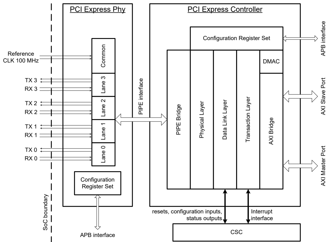
Рисунок 5.25 - Структурная схема контроллера интерфейса PCIe
