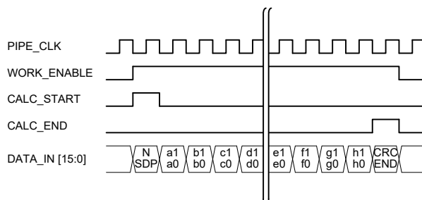
Рисунок 4.22 – Временная диаграмма работы блока генерации CRC
