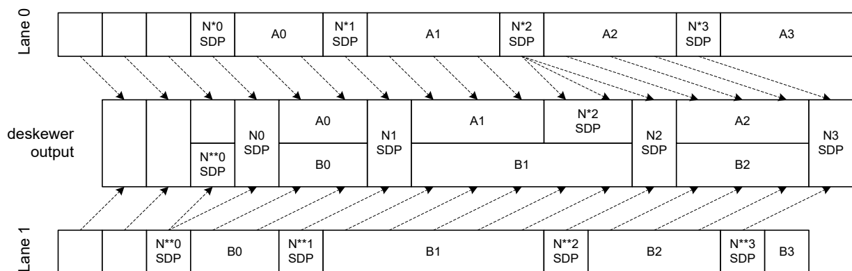
Рисунок 4.26 – Временная диаграмма работы блока DeSkewer
