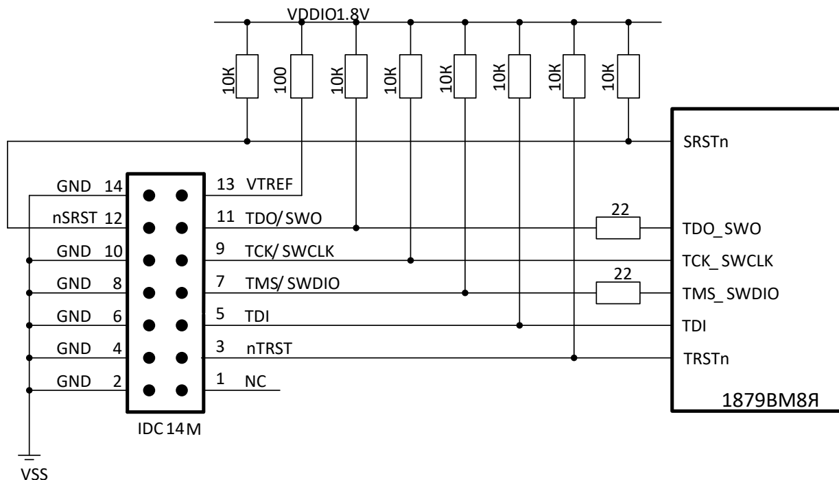
Рисунок 5.47 – Типовая схема подключения ARM JTAG 14 к микросхеме K1879BM8Я
