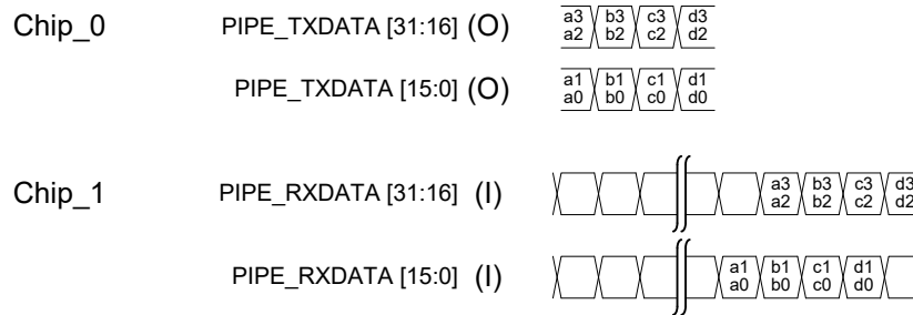
Рисунок 4.25 – Разбежка данных при передаче
