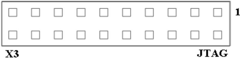
Рисунок 8 - Разъем JTAG
