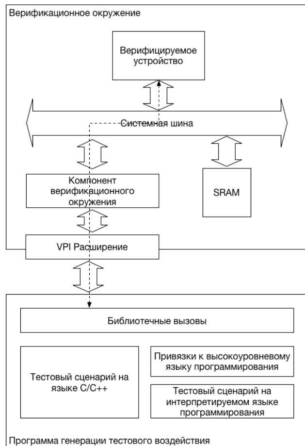
Рис. 2. Схема гибридного верификационного окружения IP блока
