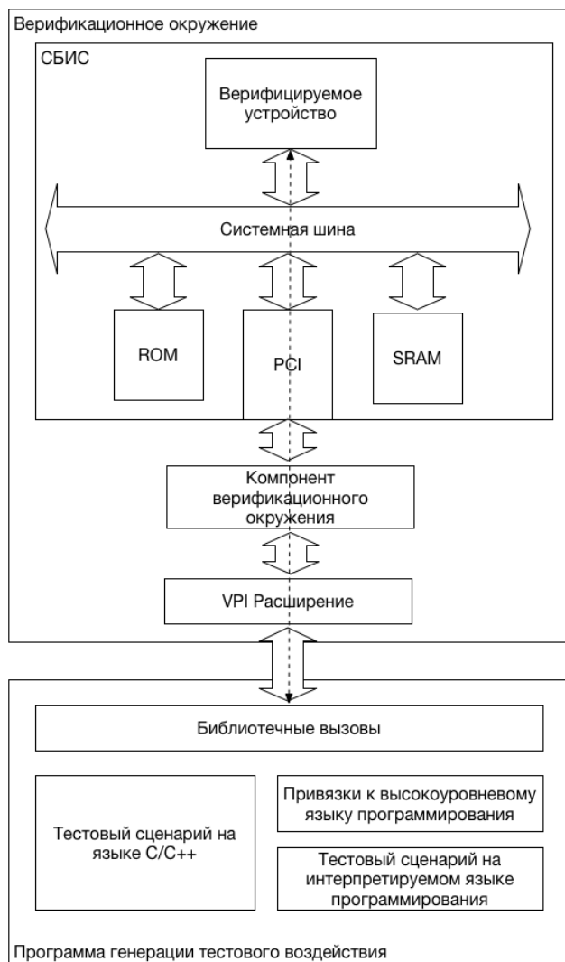
Рис. 4. Схема гибридного верификационного окружения СБИС через интерфейс PCI
