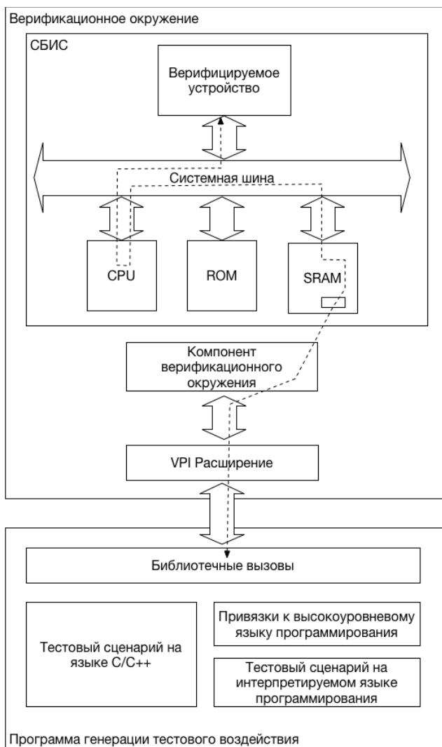
Рис. 3. Схема гибридного верификационного окружения СБИС через внутреннюю память
