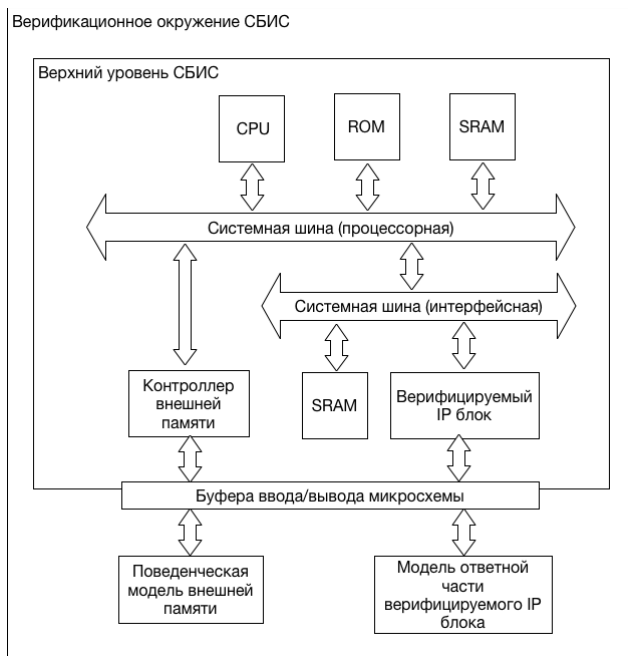
Рис. 1. Упрощенная схема верификационного окружения СБИС
